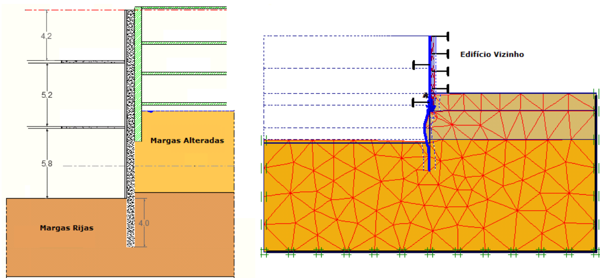
Figura 8 – Secção B (secção representativa do alçado este da obra): corte-tipo (à esquerda) e modelo de análise com a representação da deformada na última fase de escavação (à direita)
