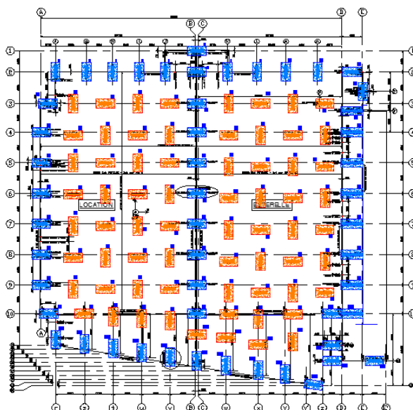
Extrait du plan d'implantation des panneaux CSM
